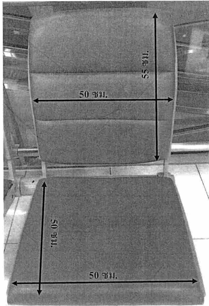
ภาพ แสดงขนาดเบาะนั่งและพนักพิงเก้าอี้โครงเหล็กชนิด 5 ที่นั่ง (2)
