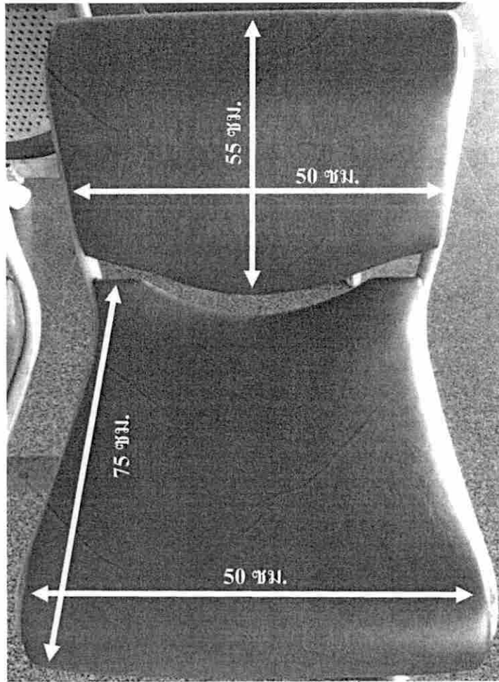
ภาพ แสดงขนาดเบาะนั่งและพนักพิงเก้าอี้ชนิด 2 ที่นั่ง (5)
