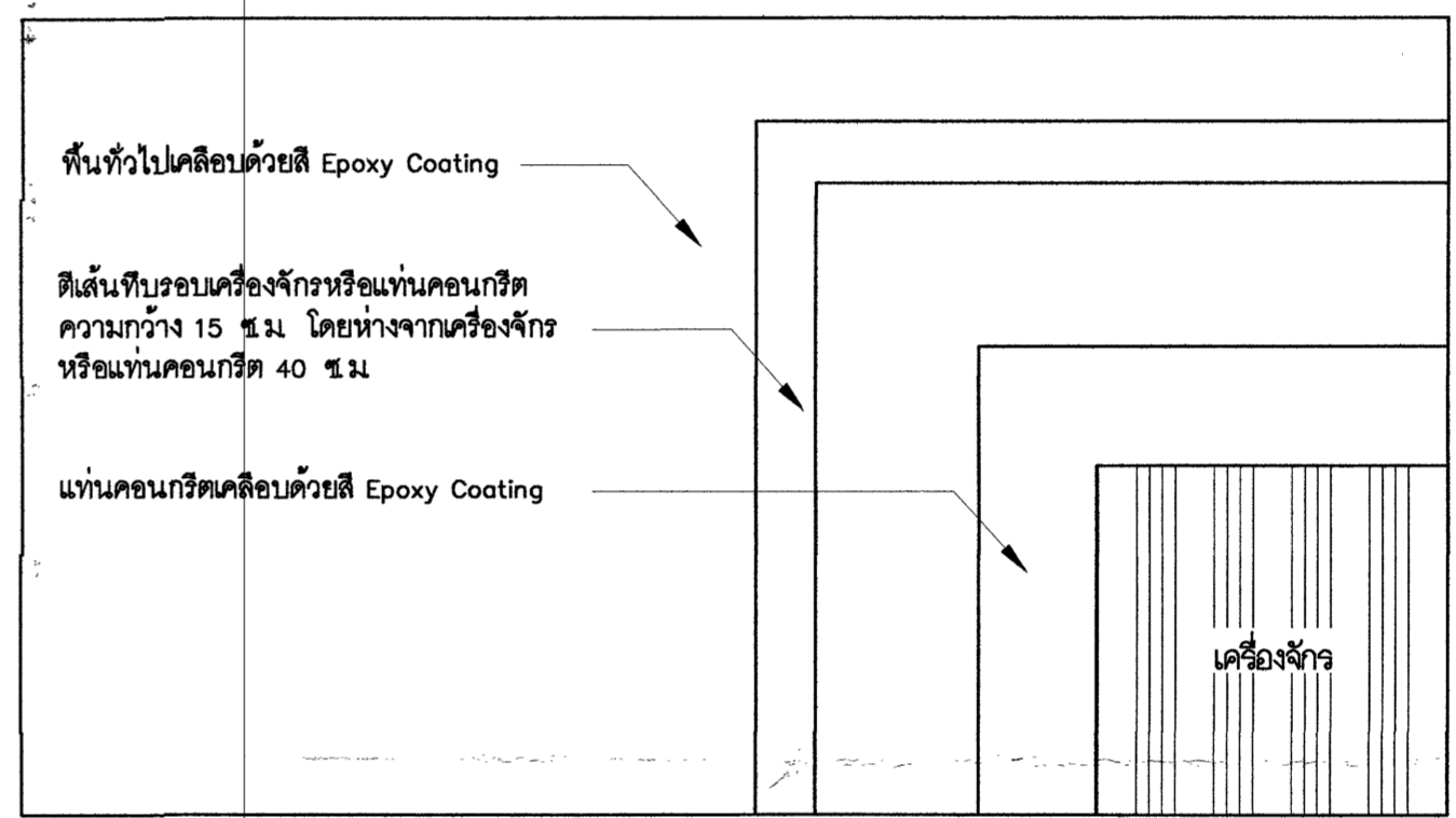
แบบขยายการเคลือบสีพื้นคอนกรีต มาตราส่วน NOT TO SCALE
