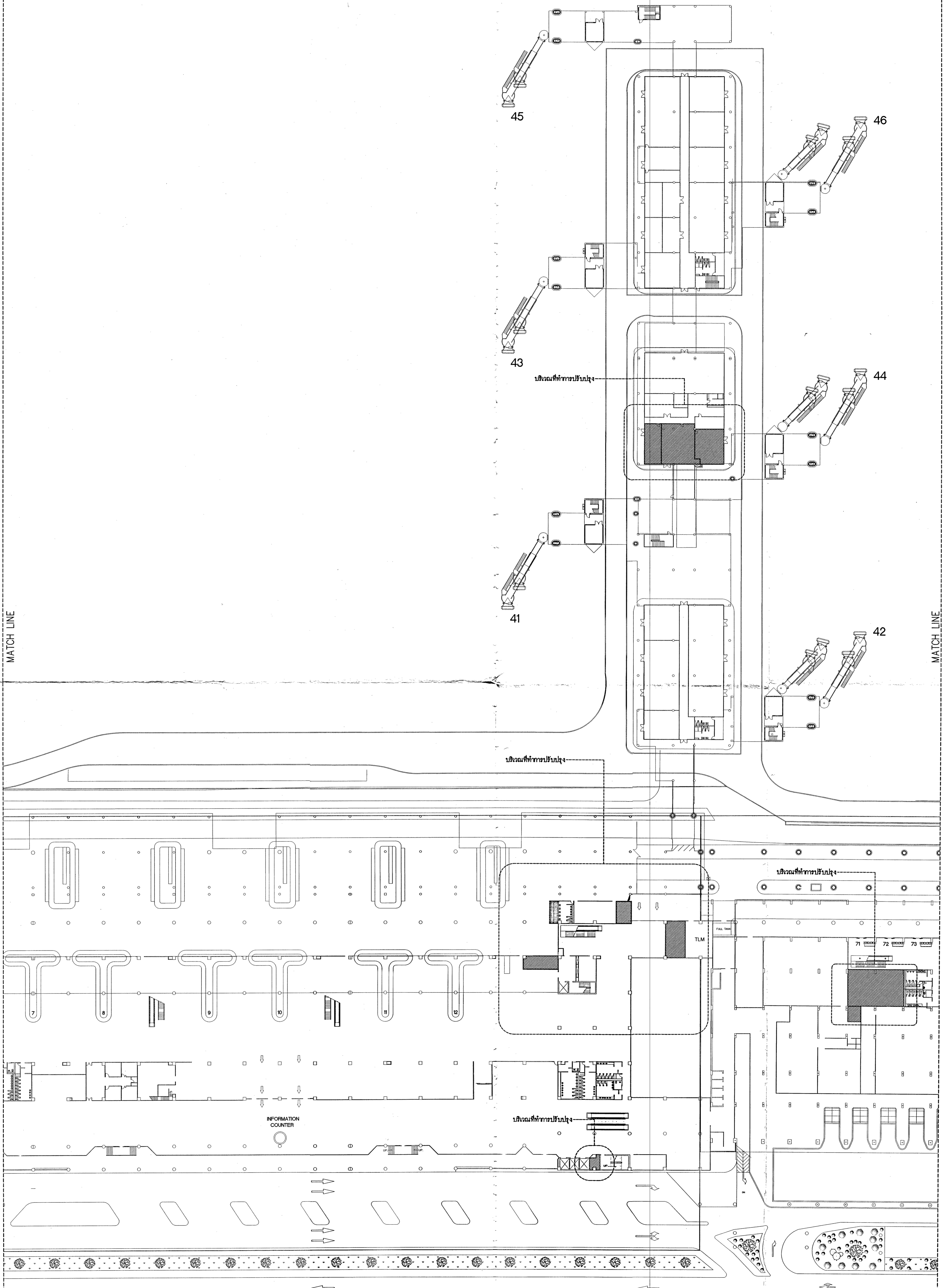
จุดตั้งที่ทำการรับกระเป๋า แบบแปลนแสดงพื้น ชั้น 1 (4/5) มาตรฐาน 1:500
