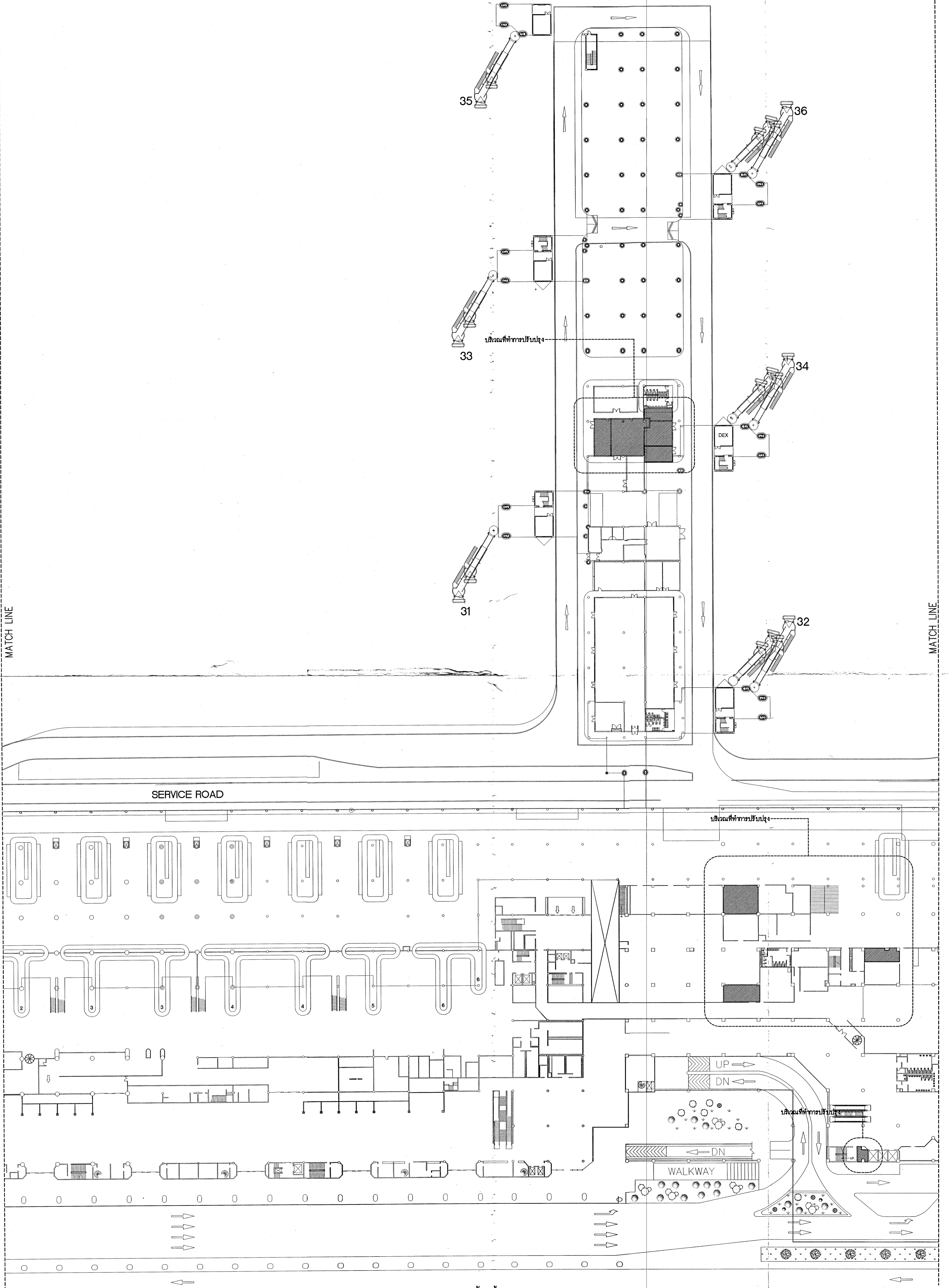
แบบแปลนแสดงพื้นที่ ชั้น 1 (3/5) มาตราส่วน 1:500
