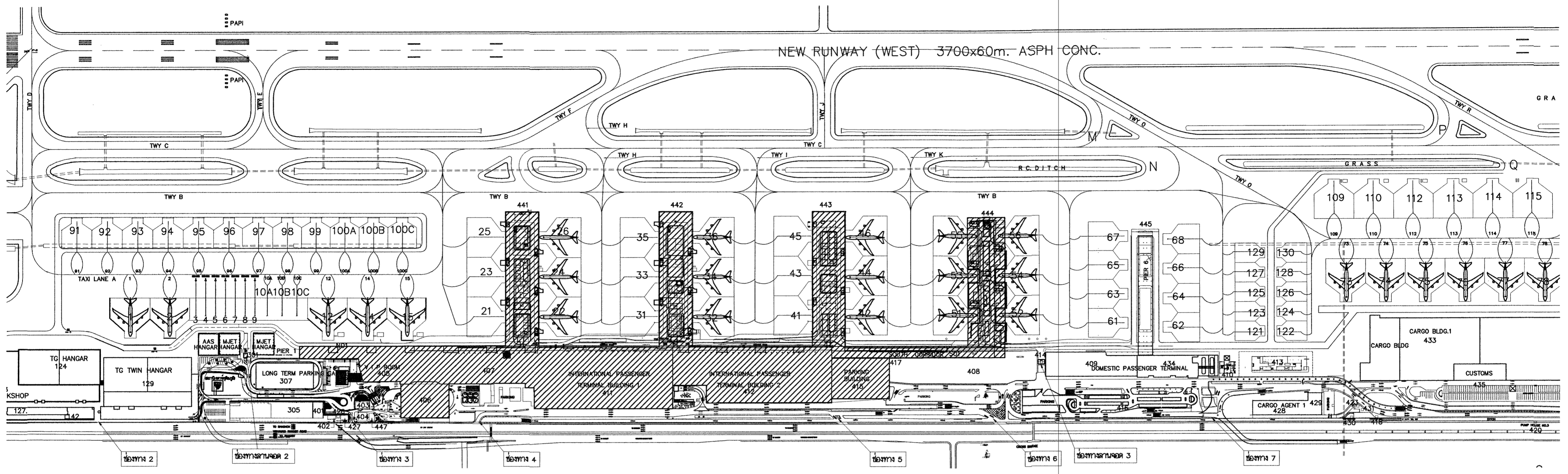
ผังบริเวณ มาตราส่วน 1:5000
