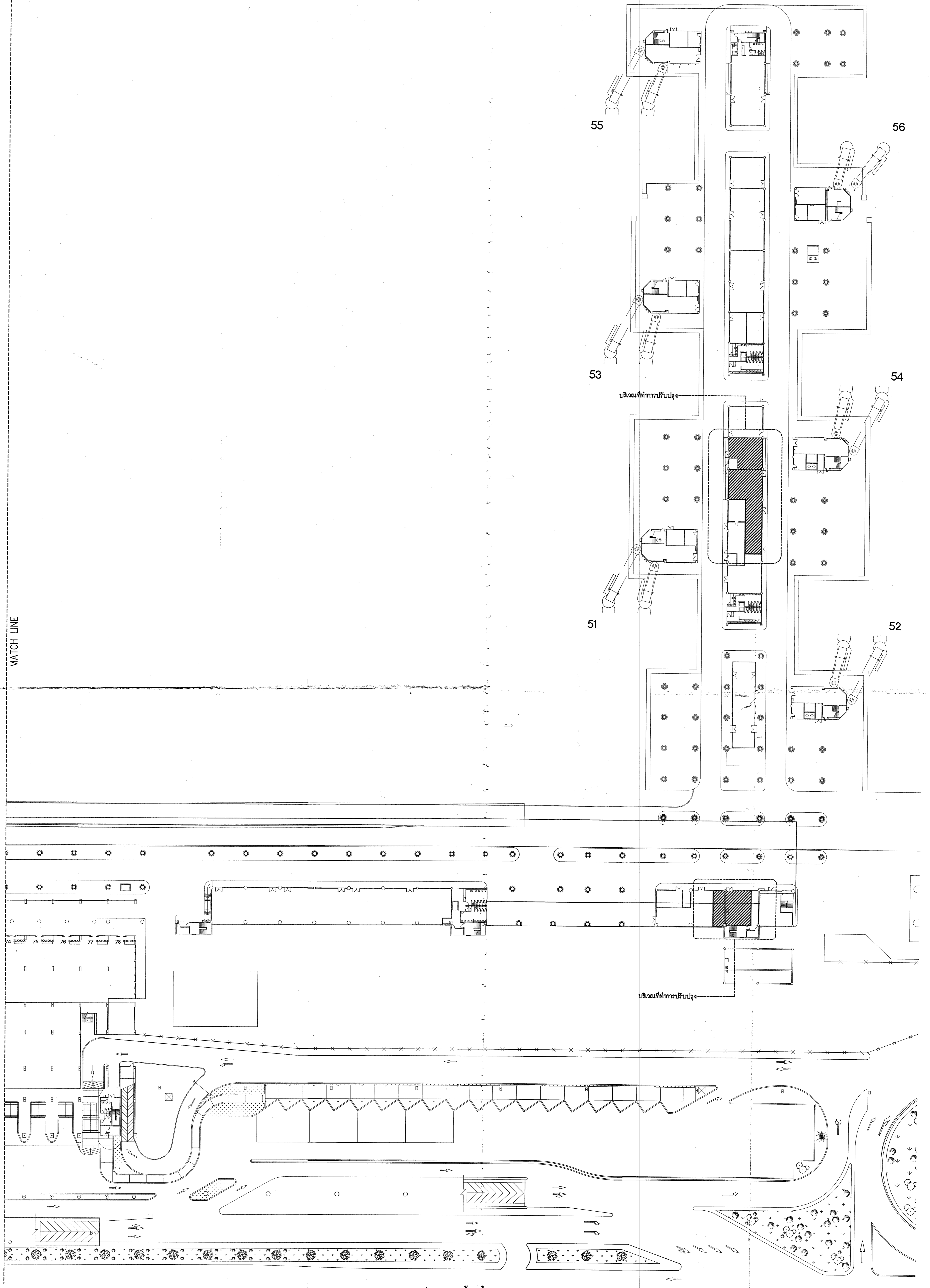
แบบแปลนแสดงพื้น ชั้น 1 (5/5) มาตรฐาน 1:500
