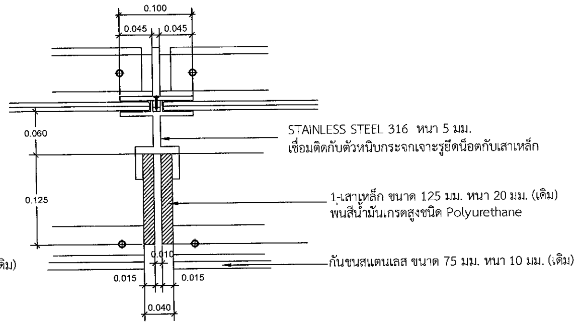
แบบขยาย (ใหม่) SCALE 1:5
