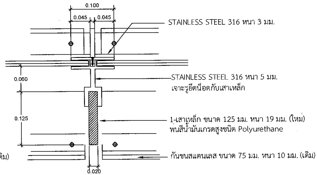
แบบขยาย (ใหม่) SCALE 1:5
