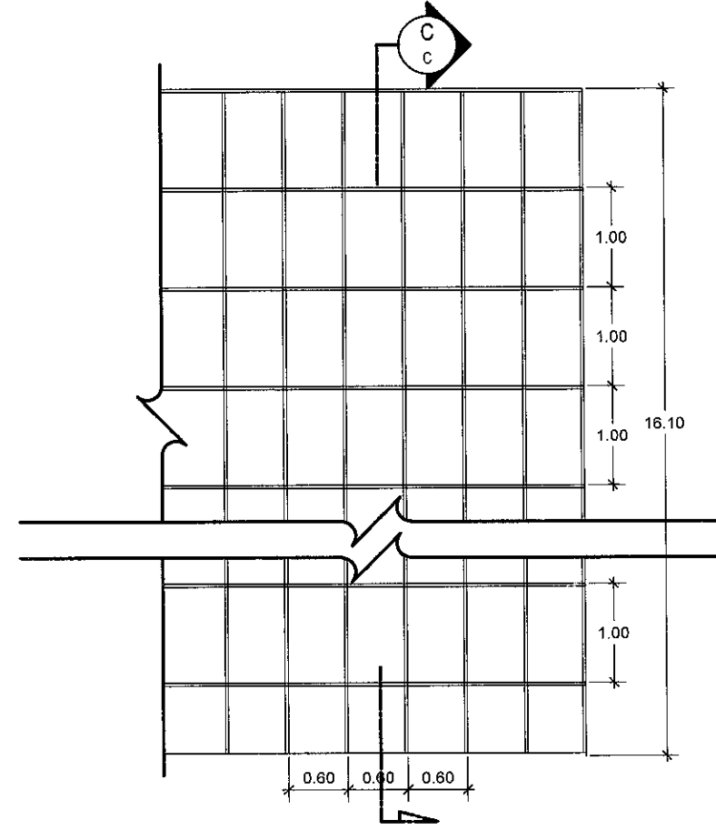
แบบขยาย 1 SCALE 1:250
