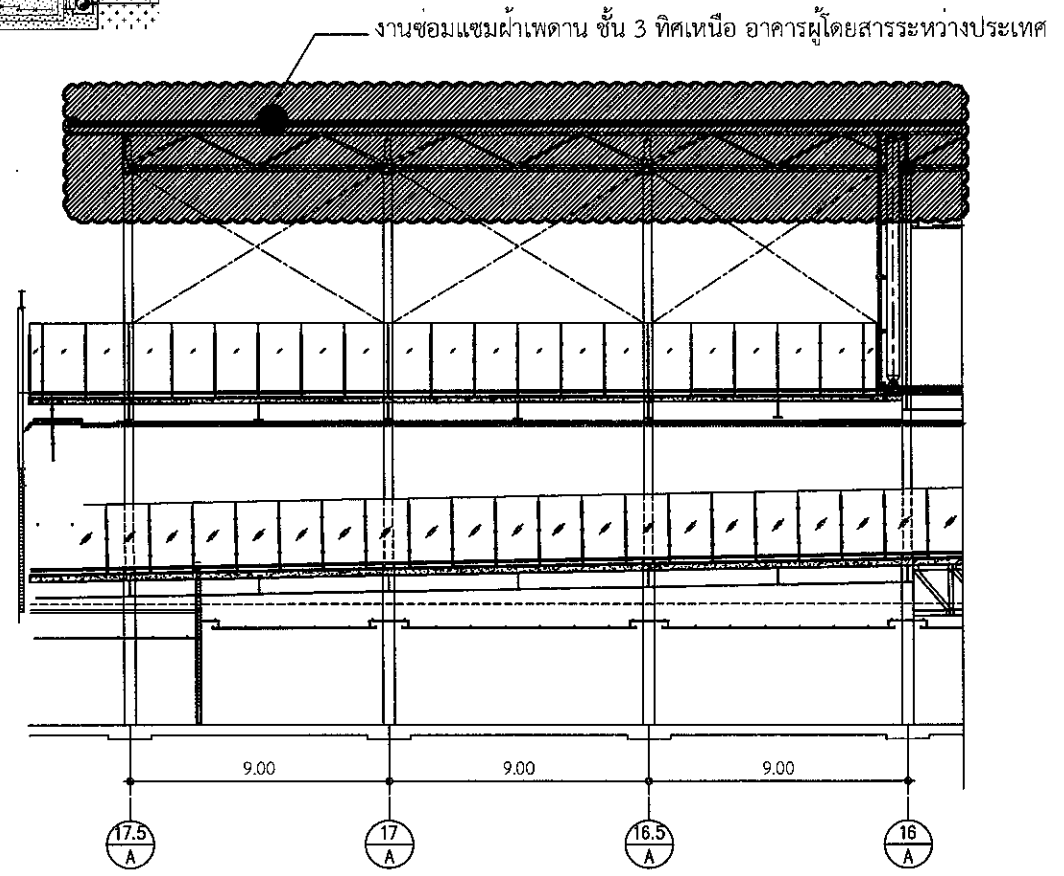
รูปตัด A SCALE 1:250
