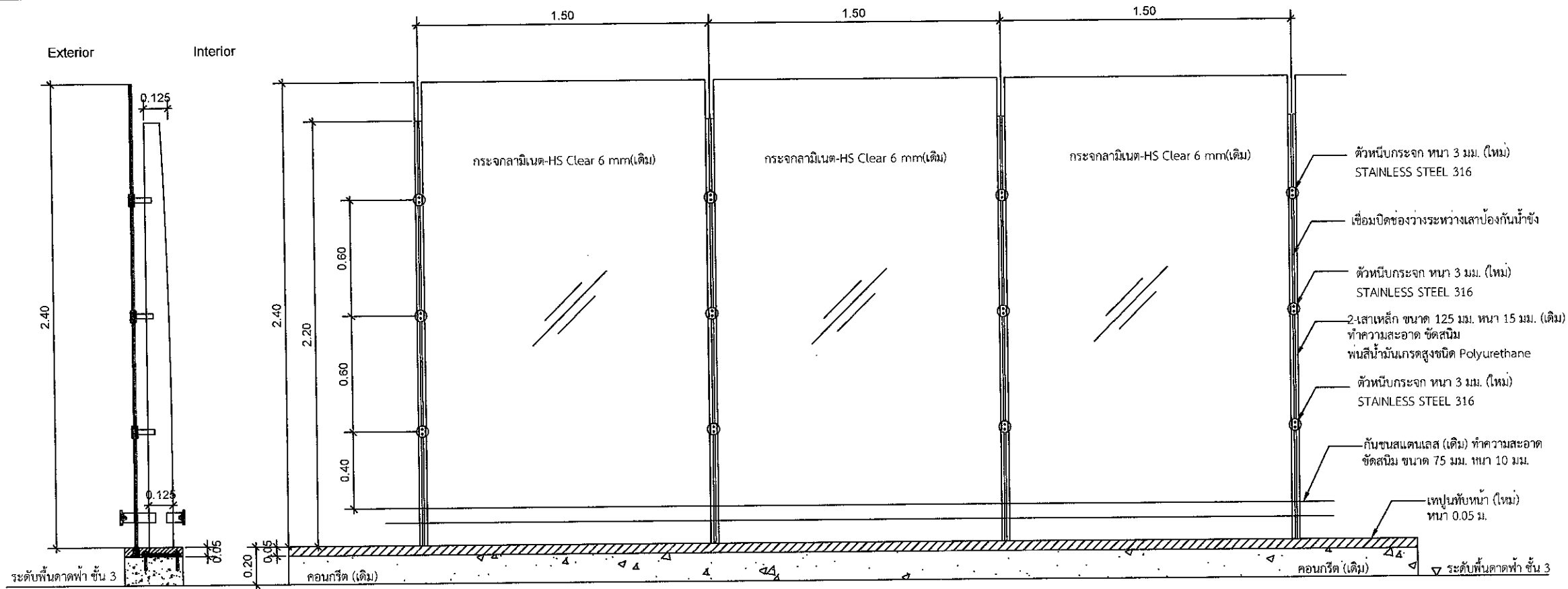
รูปด้าน 2 SCALE 1:25
