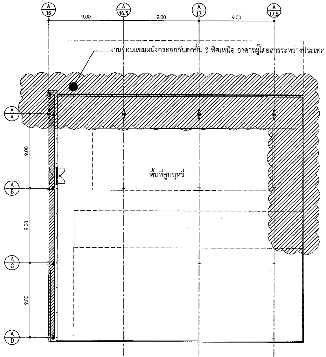
แปลนพื้น ชั้น 3 อาคารผู้โดยสารระหว่างประเทศ SCALE 1:250
