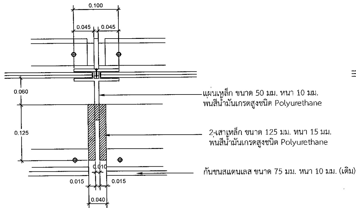
แบบขยาย (เดิม) SCALE 1:5
