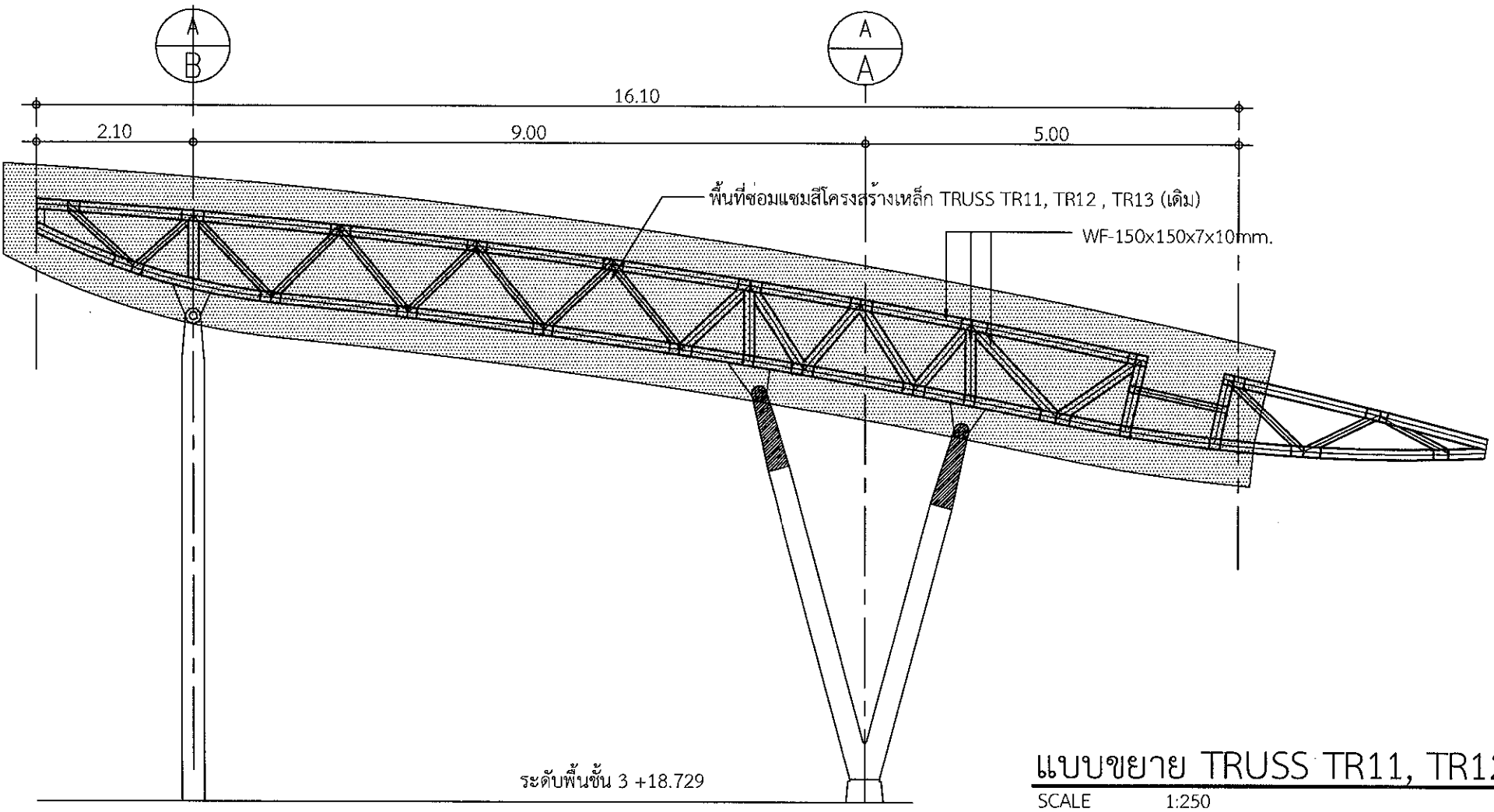
แปลนโครงสร้างค้ำ SCALE 1:250
