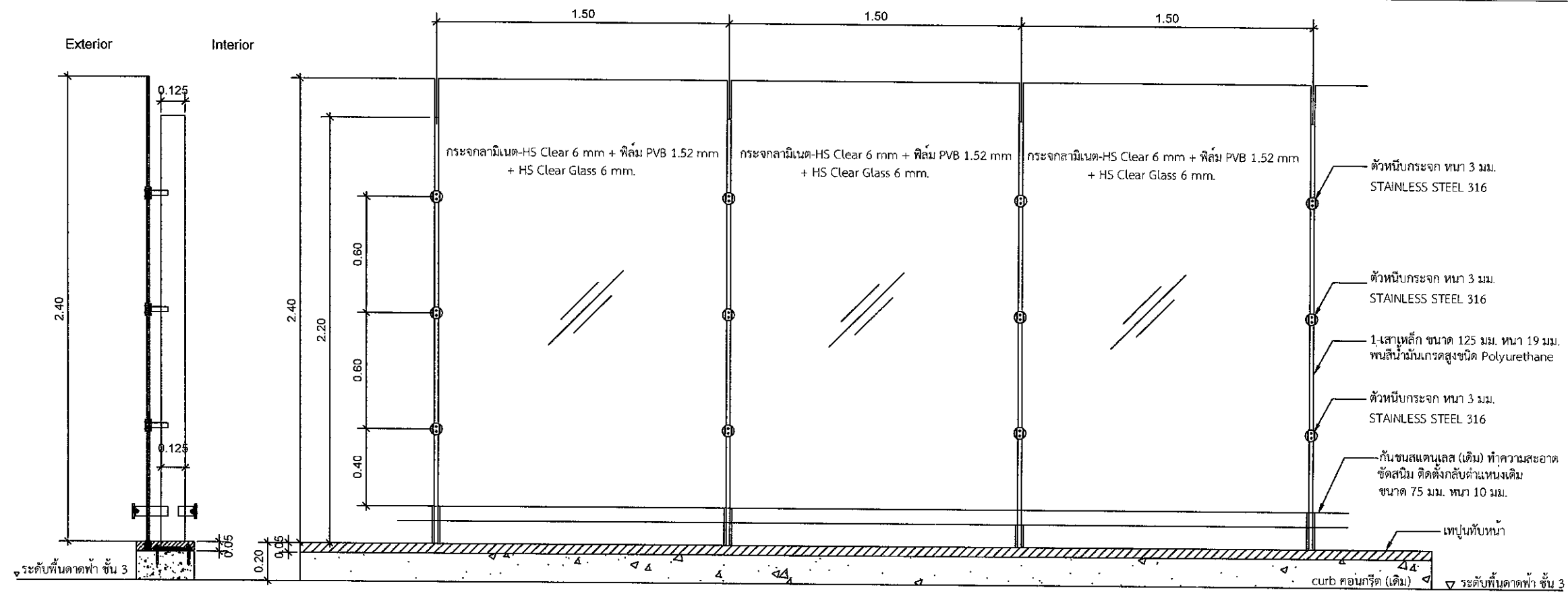
รูปด้าน 1 SCALE 1:25, 1:10
