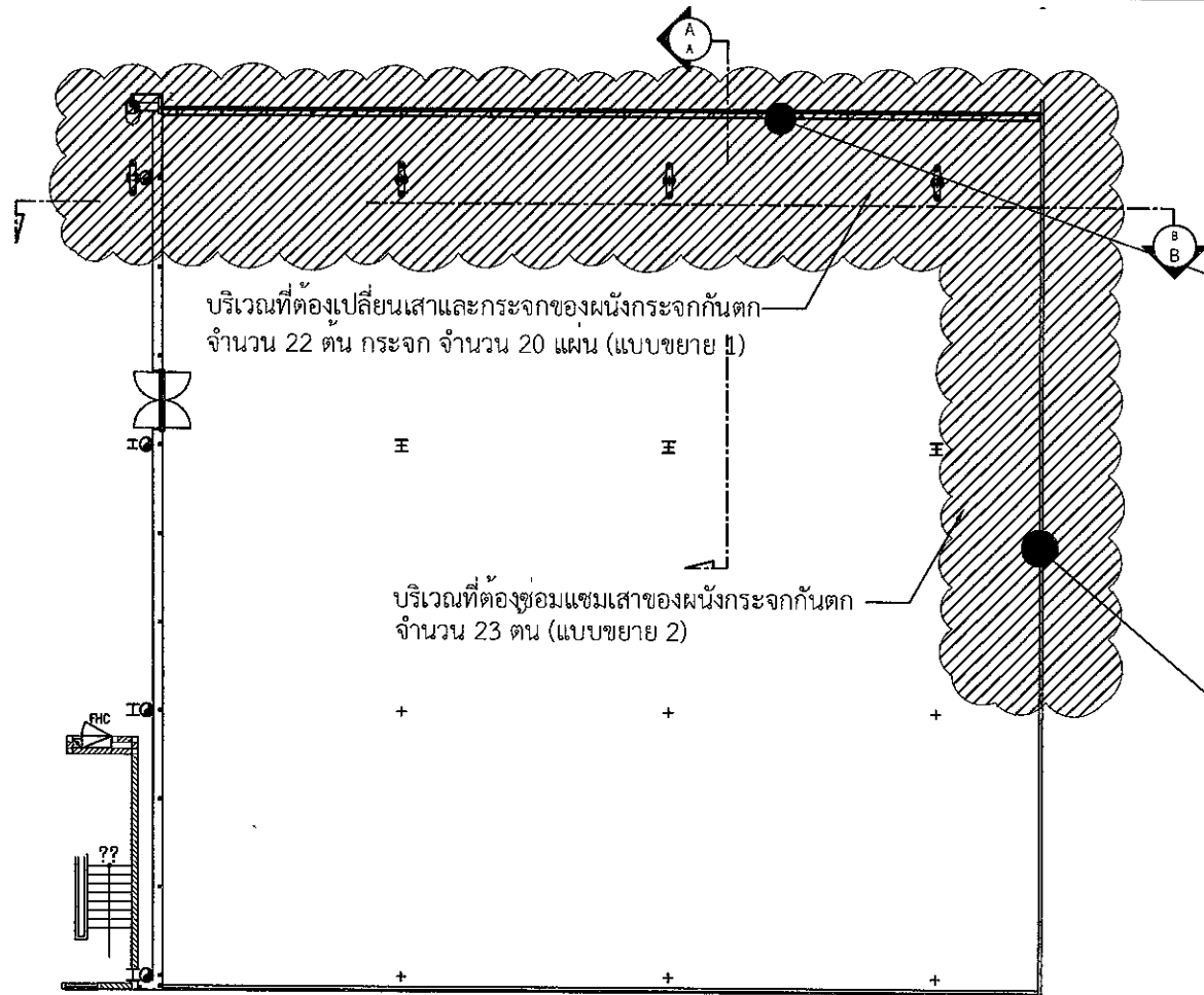
แปลนพื้น ชั้น 3 อาคารผู้โดยสารระหว่างประเทศ SCALE 1:250
