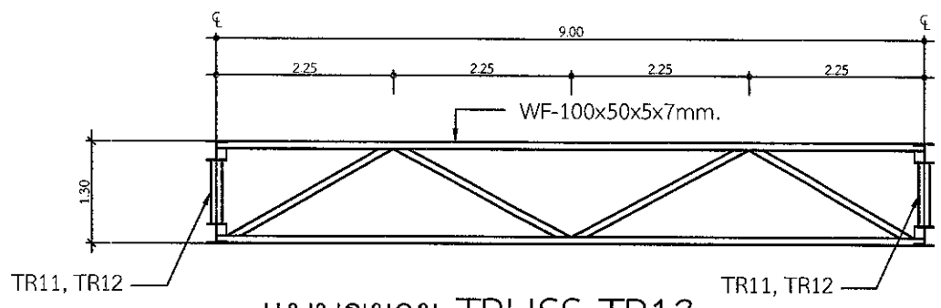
แบบขยาย TRUSS TR13 SCALE 1:150
