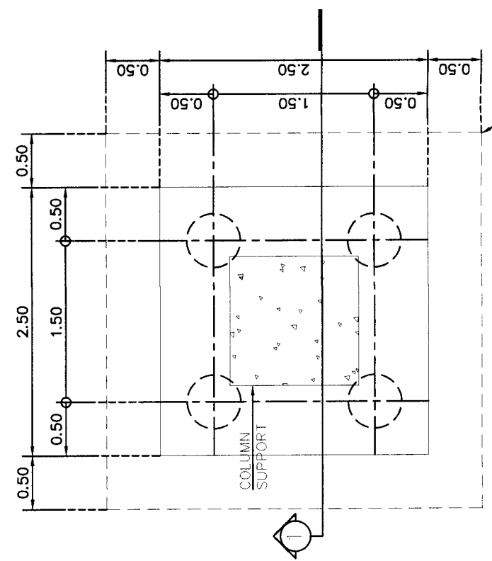
แบบขยายฐานราก 1: 50
