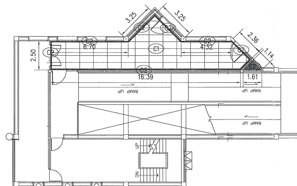
ผังผ้า GATE 24 ชั้น 2 SCALE 1:200
