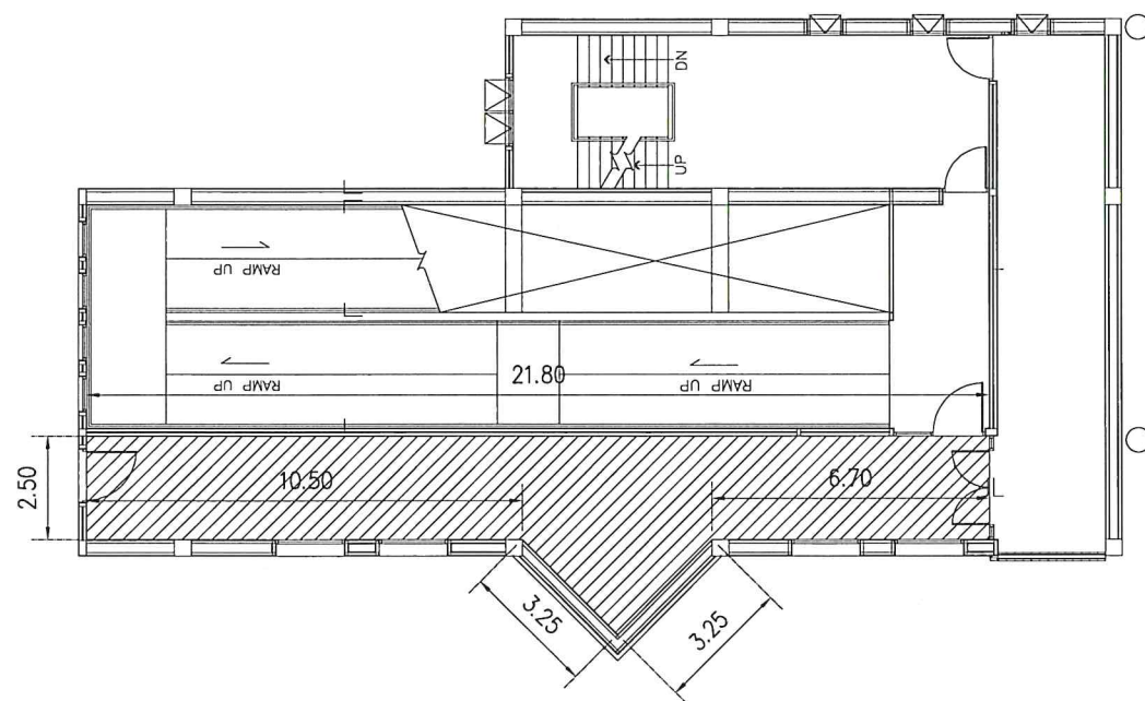
ฝ้ารื้อถอนฝ้า GATE 21 ชั้น 2
