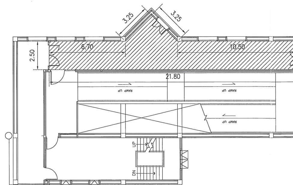
ผังรื้อถอนผ้า GATE 44 ชั้น 2 SCALE 1:200
