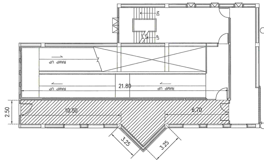
ฝั่งรื้อถอนฝ้า GATE 33 ชั้น 2
