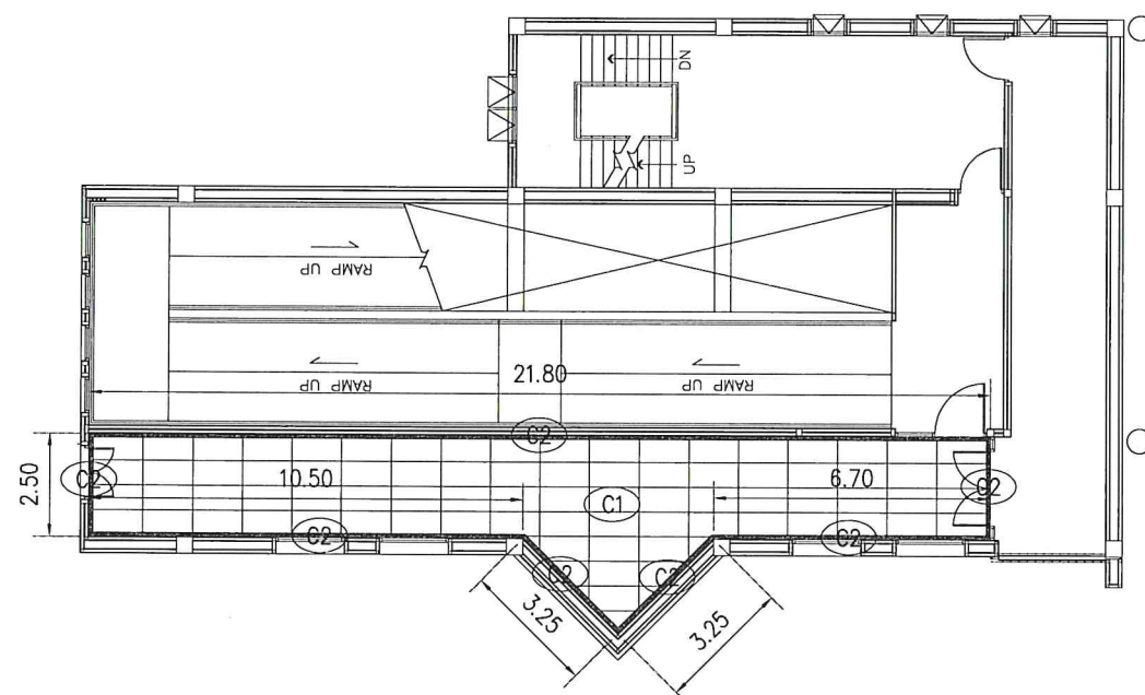
ฝ้าฝ้า GATE 41 ชั้น 2 SCALE 1:200
