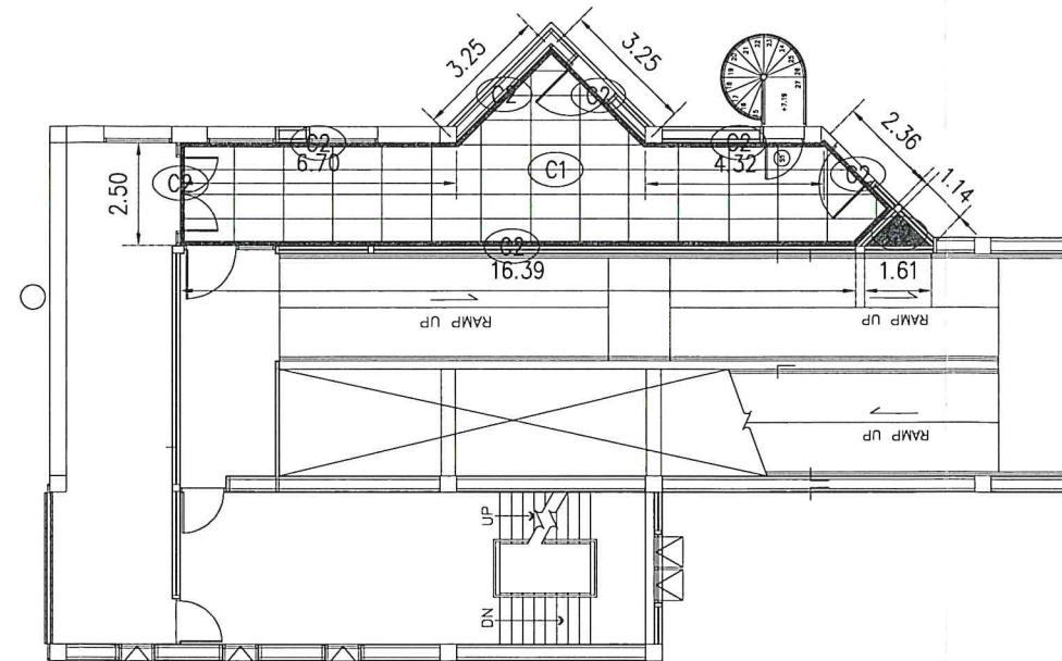
ผังผ้า GATE 22 ชั้น 2 SCALE 1:200
