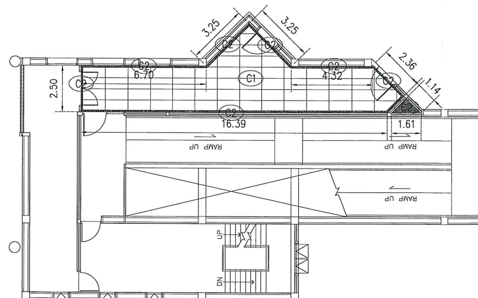
ฝ้าฝ้า GATE 36 ชั้น 2
