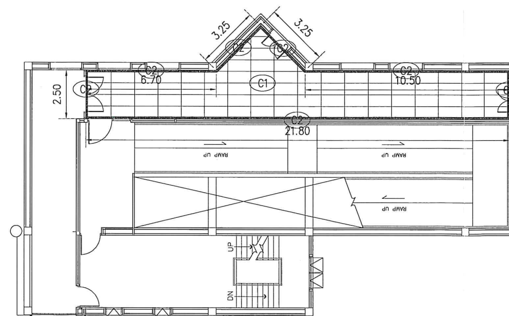
ฝ้าฝ้า GATE 44 ชั้น 2 SCALE 1:200
