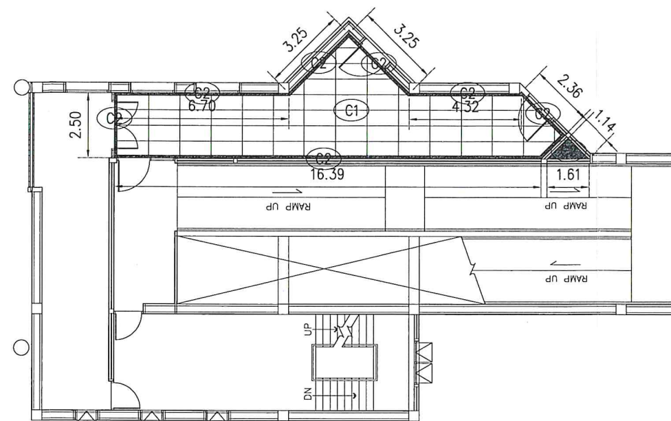
ฝั่งฟ้า GATE 26 ชั้น 2 SCALE 1:200
