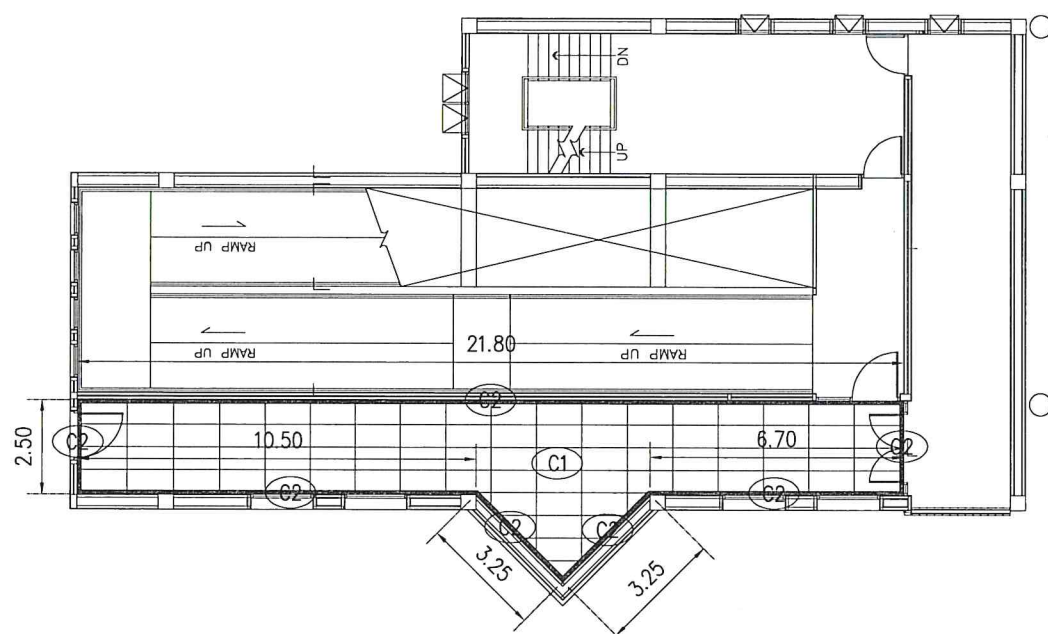
ผังผ้า GATE 21 ชั้น 2 SCALE 1:200
