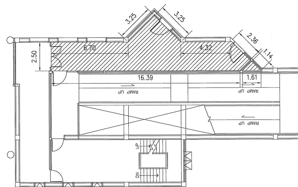
ฝั่งรื้อถอนฝ้า GATE 36 ชั้น 2
