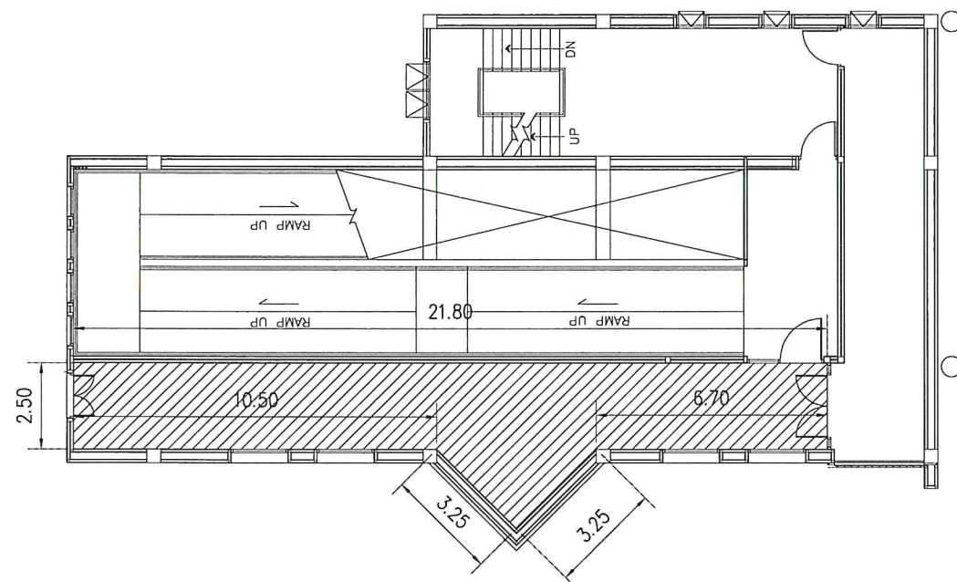
ผังรื้อถอนผ้า GATE 41 ชั้น 2 SCALE 1:200
