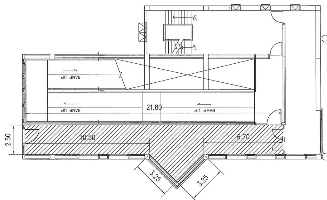
ฝ้ารื้อถอนฝ้า GATE 23 ชั้น 2
