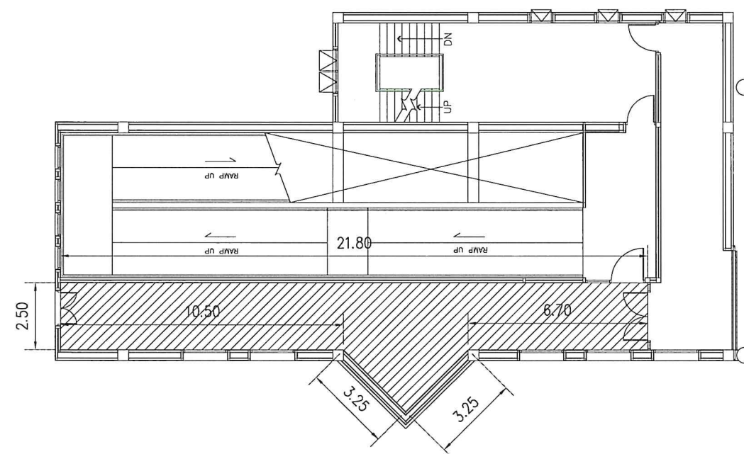
ผังรื้อถอนผ้า GATE 43 ชั้น 2 SCALE 1:200
