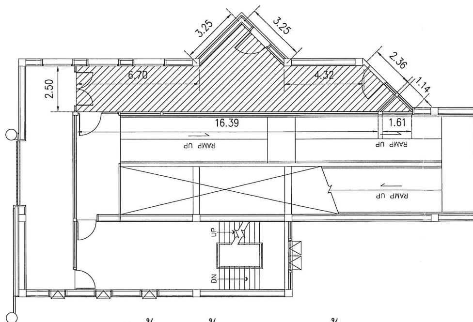
ฝั่งรื้อถอนฝ้า GATE 32 ชั้น 2
