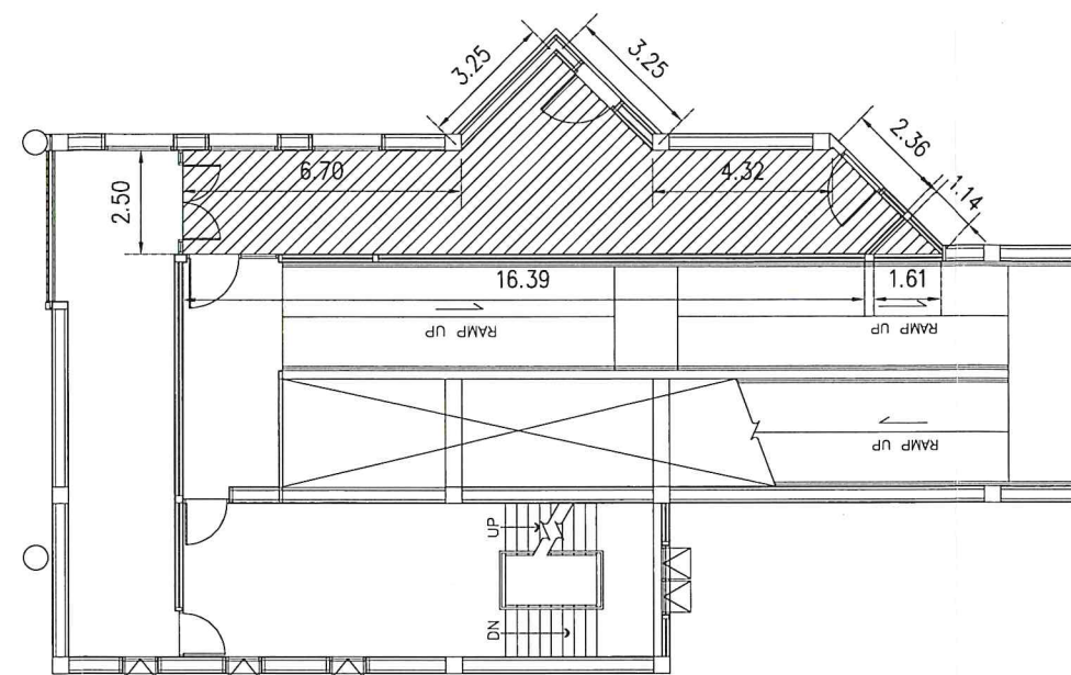
ฝั่งรื้อถอนฝ้า GATE 26 ชั้น 2
