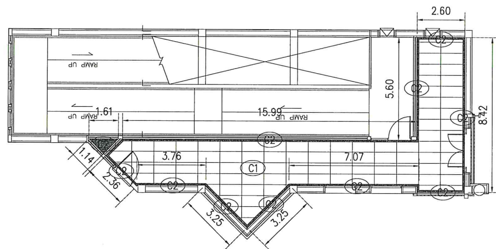
ฝั่งฟ้า GATE 25 ชั้น 2 SCALE 1:200
