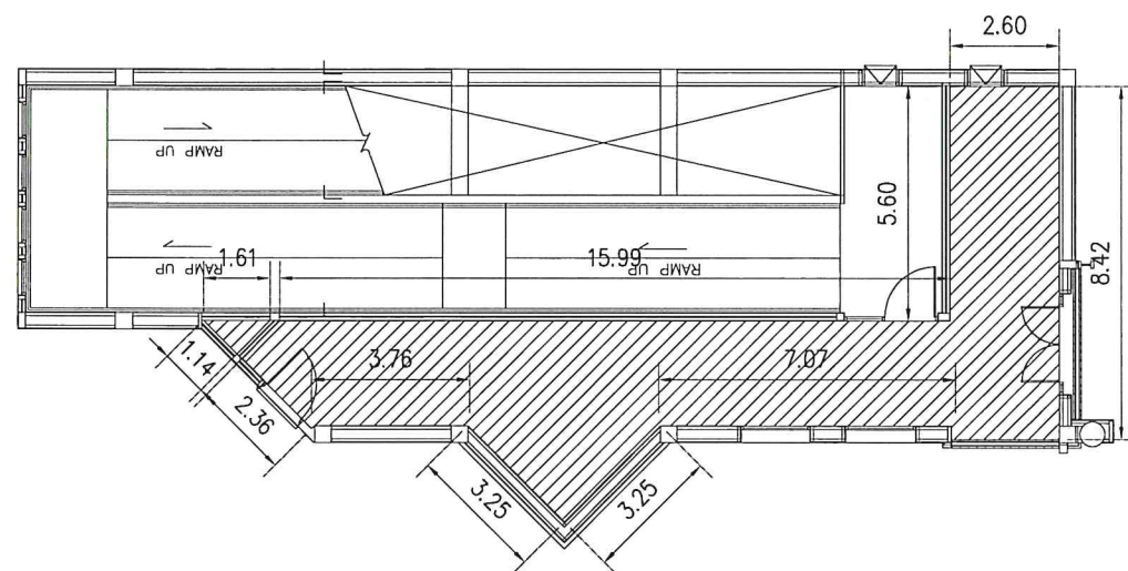
ฝั่งรื้อถอนฝ้า GATE 25 ชั้น 2
