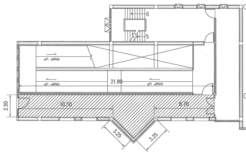
ฝั่งรื้อถอนฝ้า GATE 31 ชั้น 2
