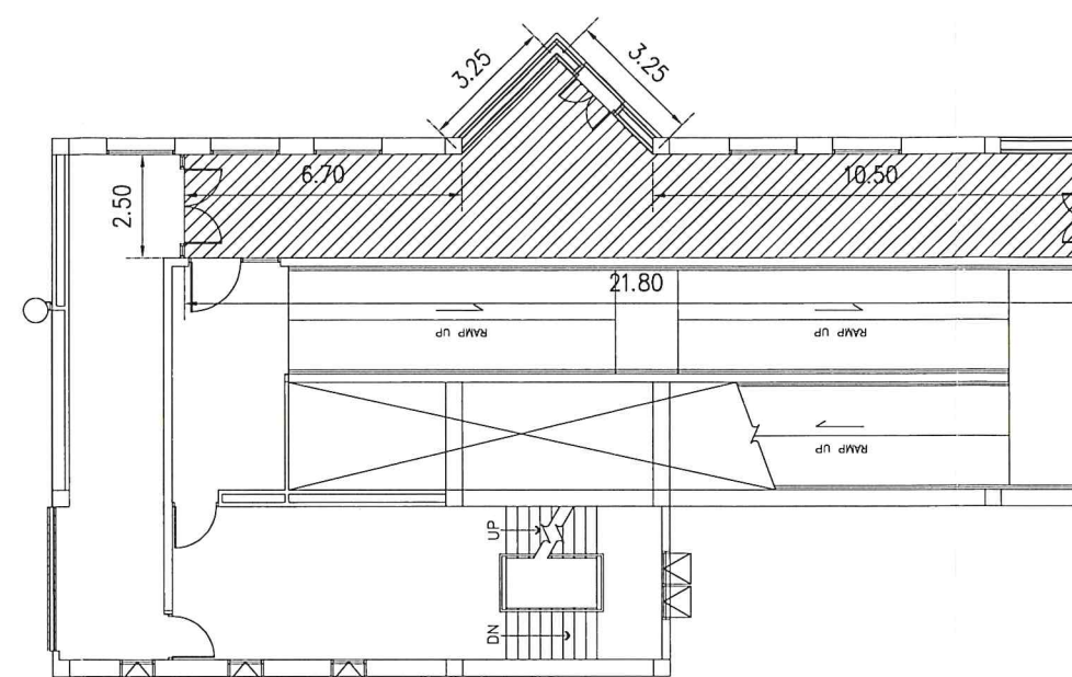
ผังรื้อถอนผ้า GATE 42 ชั้น 2 SCALE 1:200
