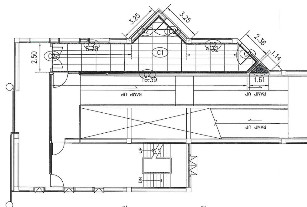
ฝั่งฟ้า GATE 32 ชั้น 2 SCALE 1:200
