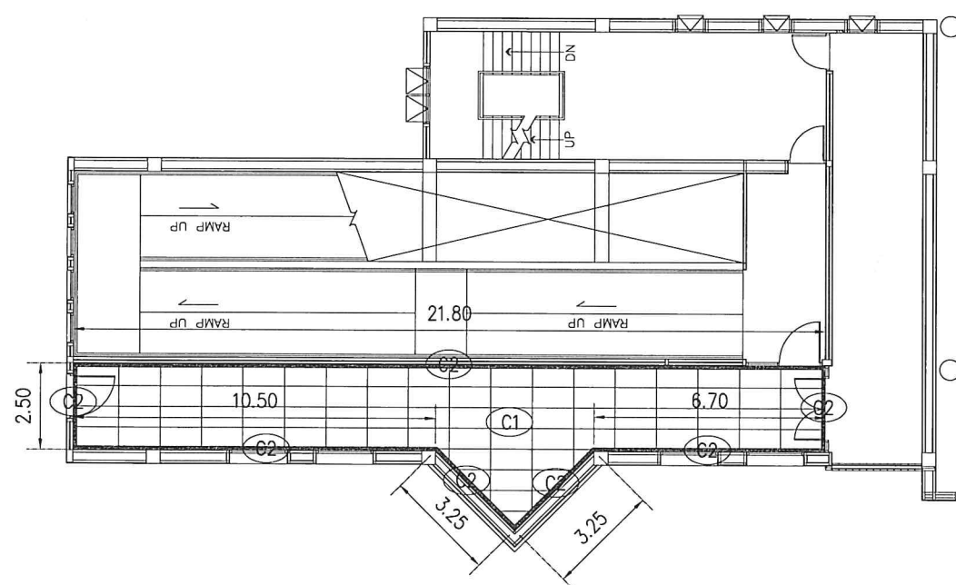
ฝั่งฟ้า GATE 31 ชั้น 2 SCALE 1:200
