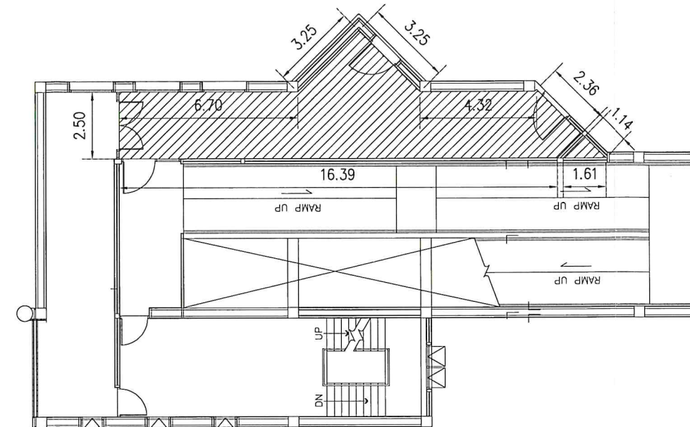
ฝั่งรื้อถอนฝ้า GATE 34 ชั้น 2
