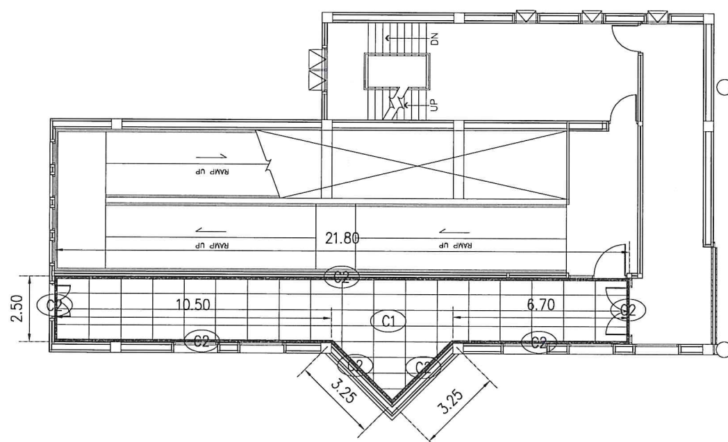
ฝ้าฝ้า GATE 43 ชั้น 2 SCALE 1:200
