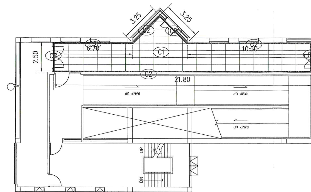
ฝ้าฝ้า GATE 42 ชั้น 2 SCALE 1:200
