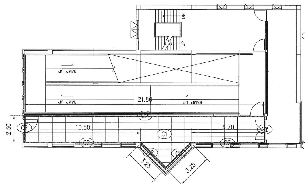
ผังผ้า GATE 23 ชั้น 2 SCALE 1:200
