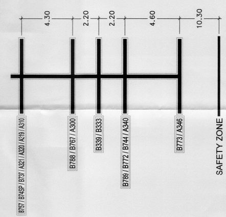
APRON NO.81
