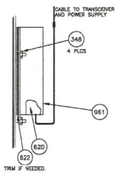
VIEW A-A
