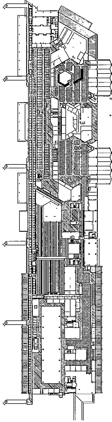
ผังฝ้าอาคารผู้โดยสารท่าอากาศยานเชียงใหม่ ชั้นที่ 2
