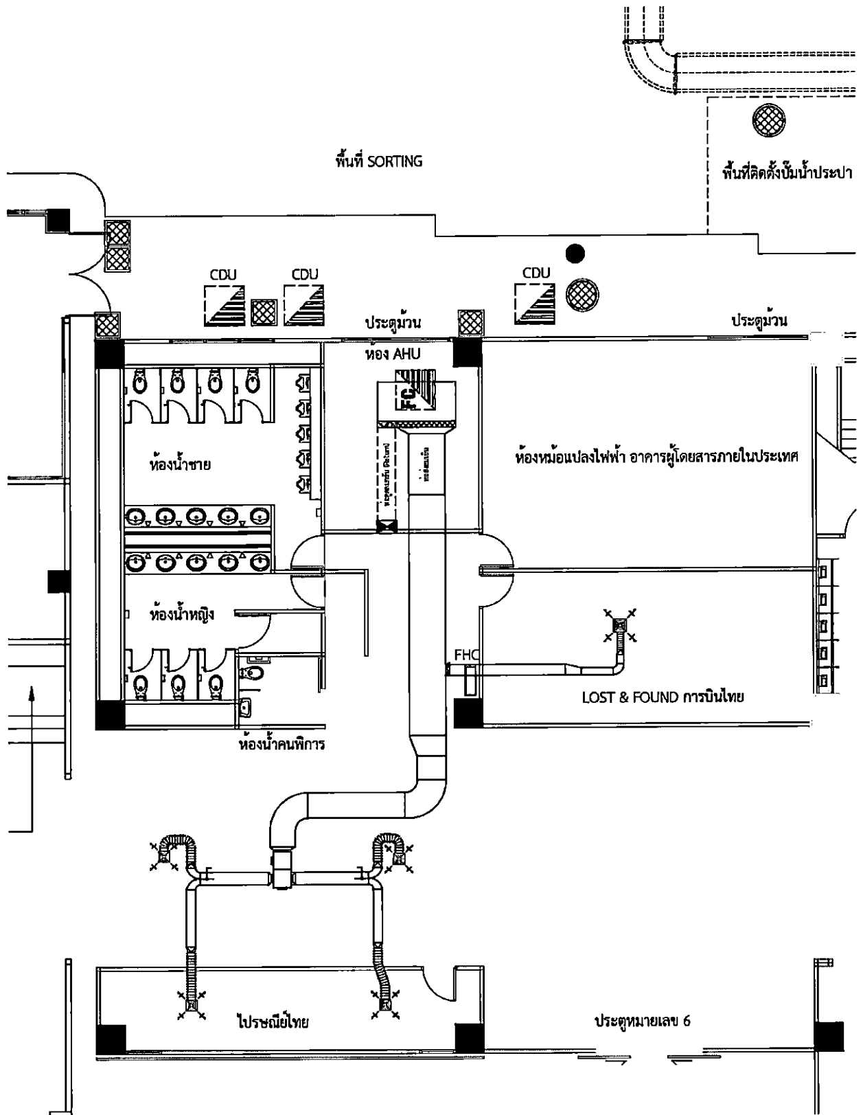
ผัง EXISTING ระบบปรับอากาศ (FCU เดิม)
